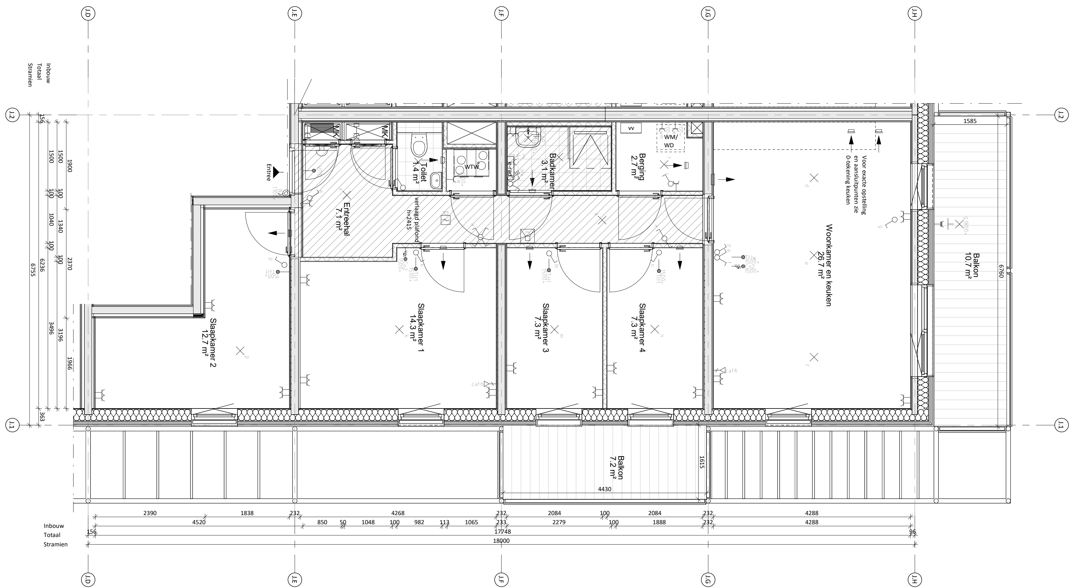
Woningtype J24 1 : 50
