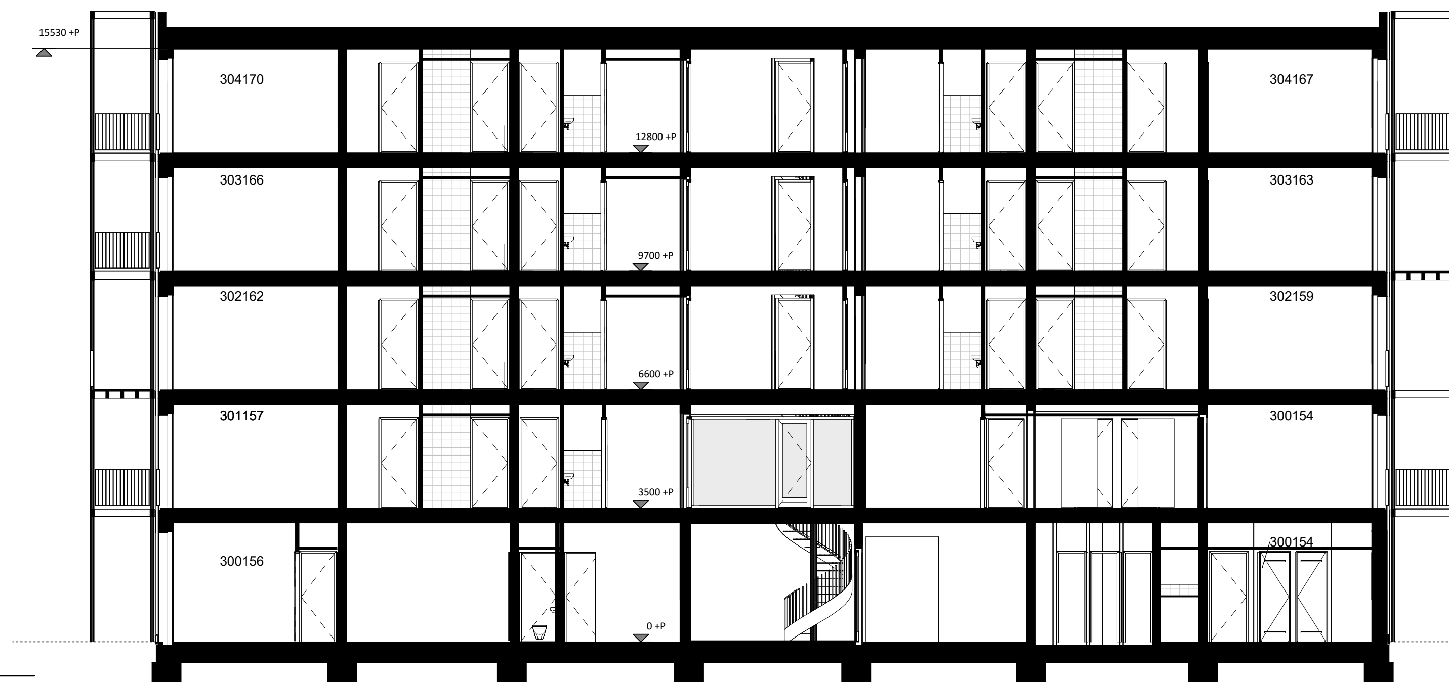
Doorsnede 1 : 100
