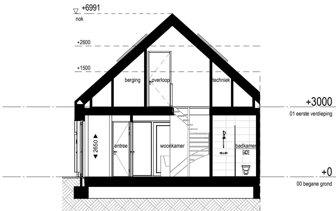
Doorsnede A 1 : 100
