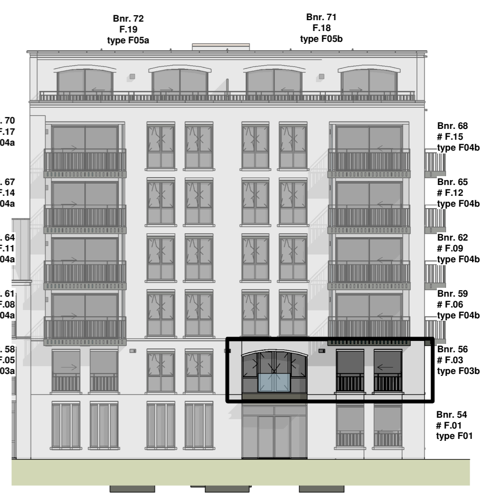
blok F - voorgevel
