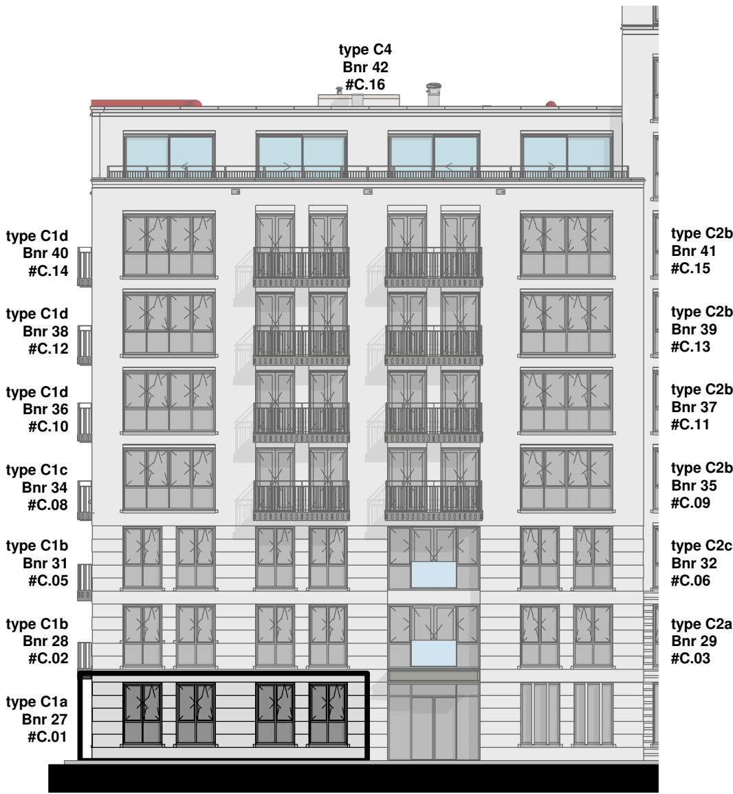
blok C - voorgevel
