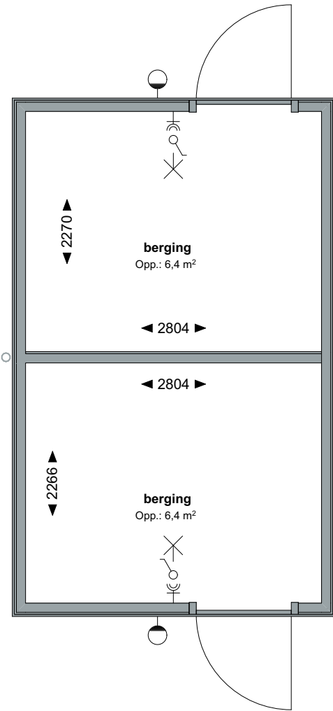
Begane grond 1:50
