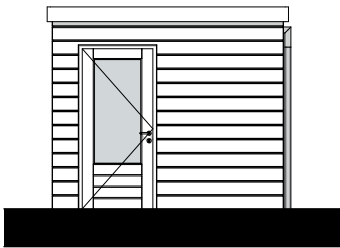
Linkergevel 1:100
