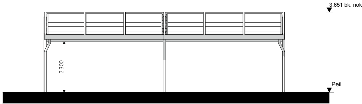
Voorgevel
