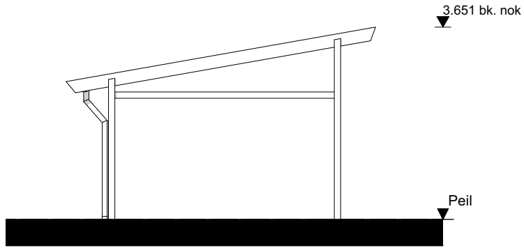
Rechtergevel
