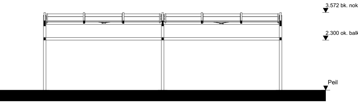
Doorsnede A-A
