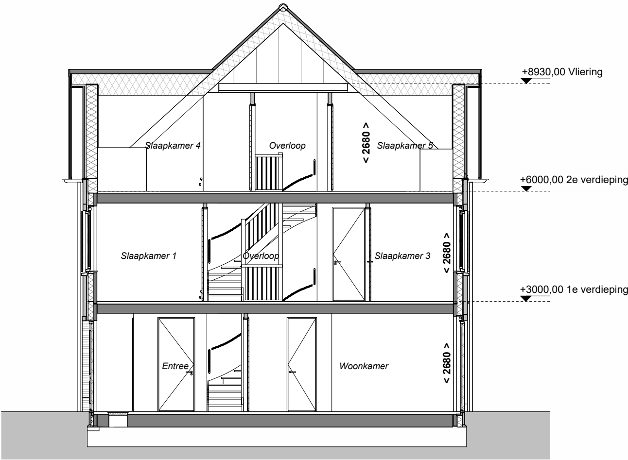
Doorsnede
