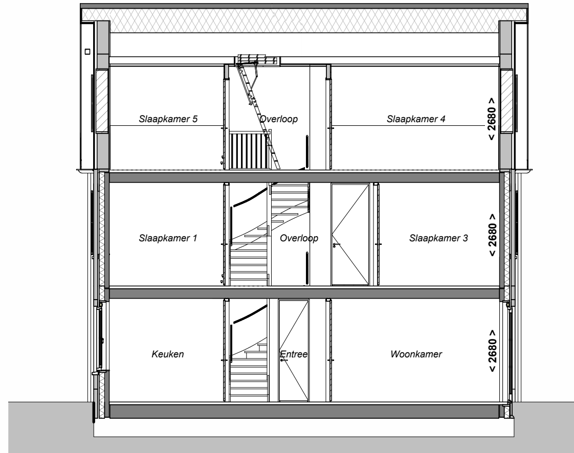
Doorsnede A-A
