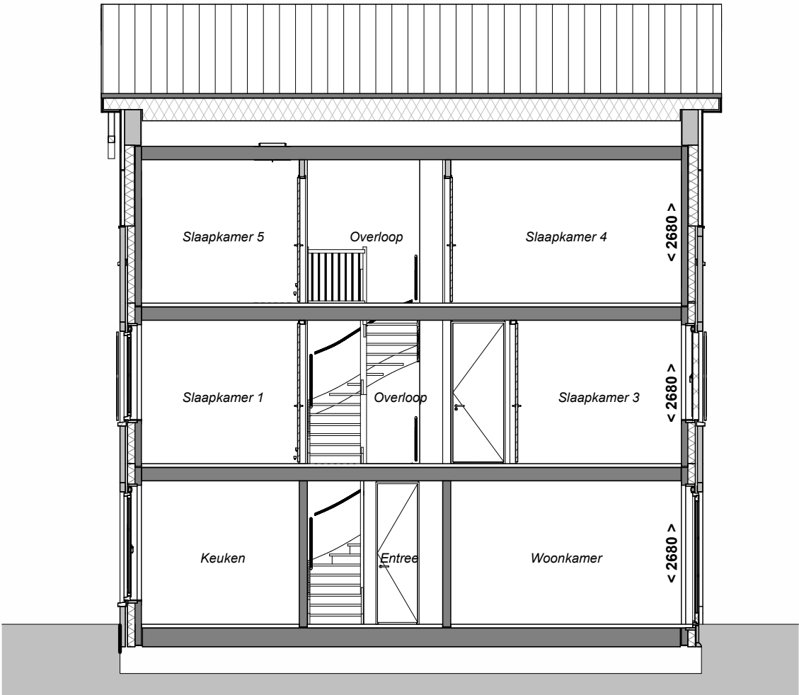
Doorsnede A-A
