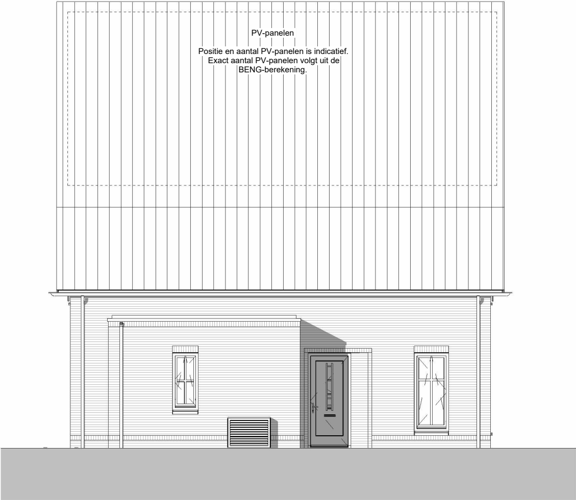
Linkergevel
