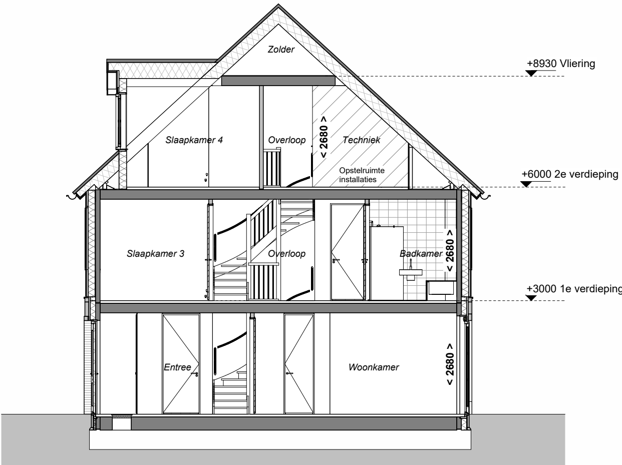
Doorsnede
