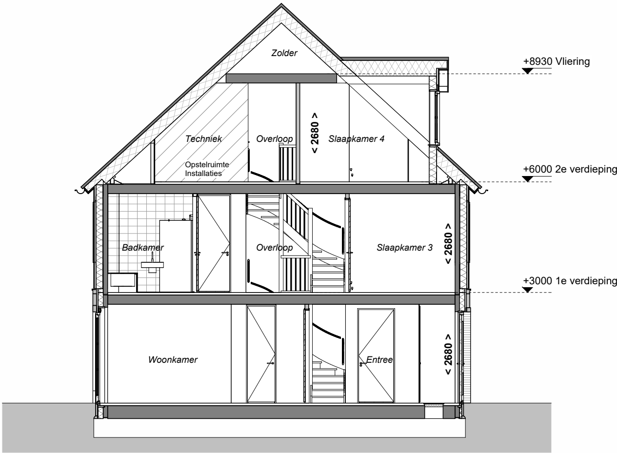
Doorsnede
