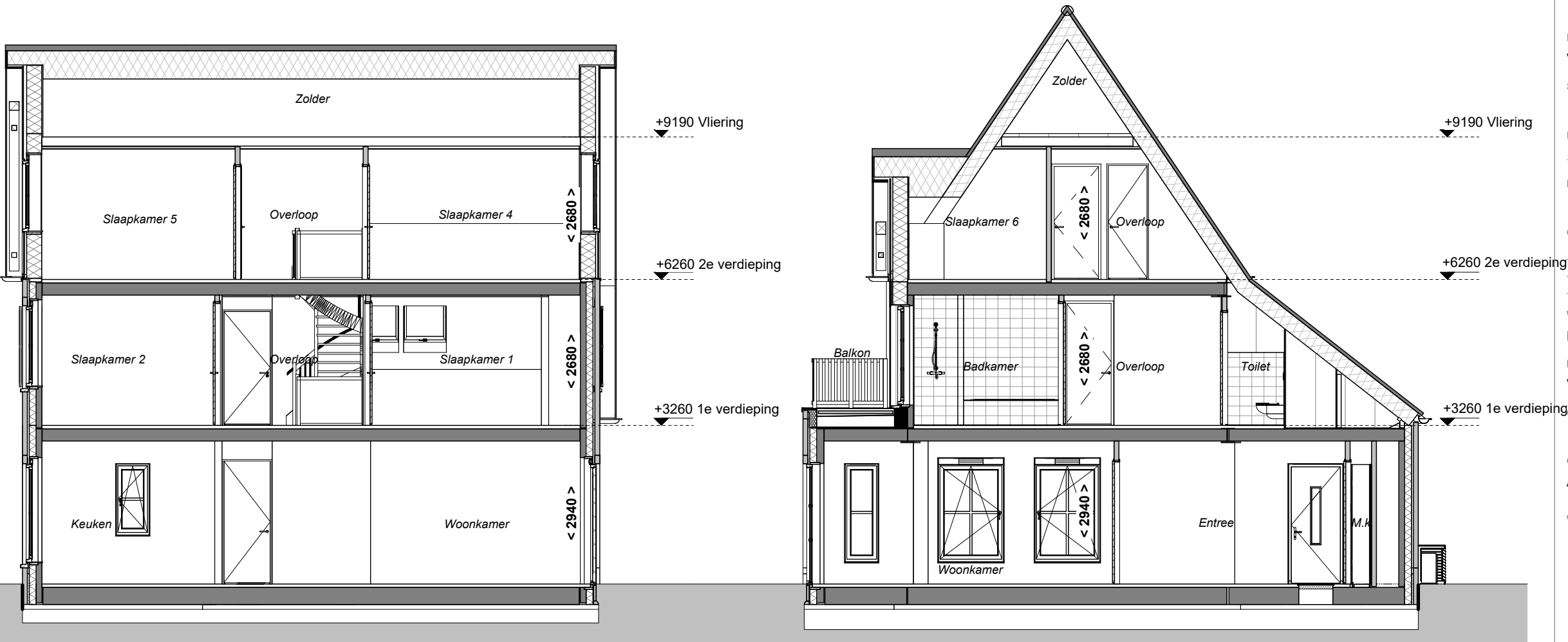
Doorsnede B-B
