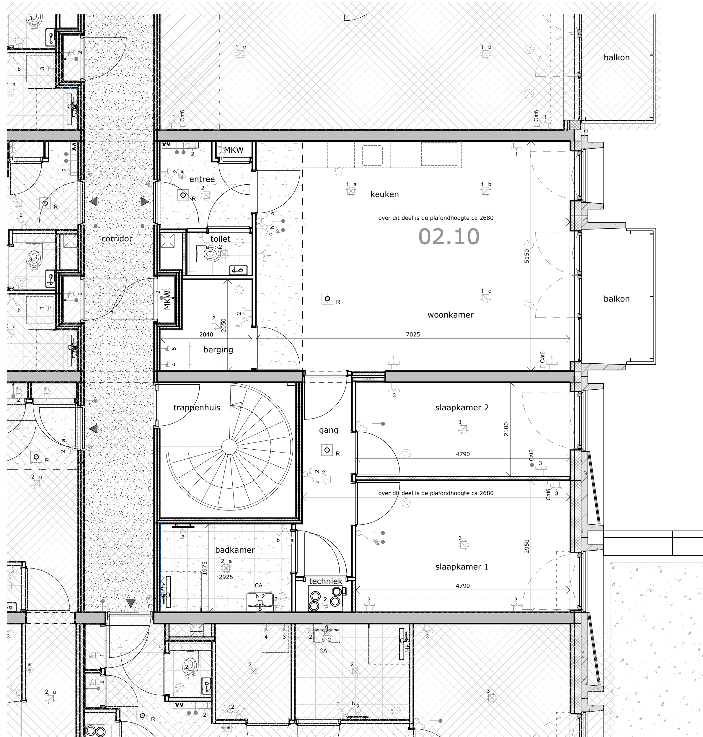
plattegrond bouwnummer 02.10 (tweede verdieping) schaal 1 : 50
